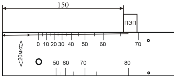
СО-2 (или СО-3Р) N СО-2 , ДБ
